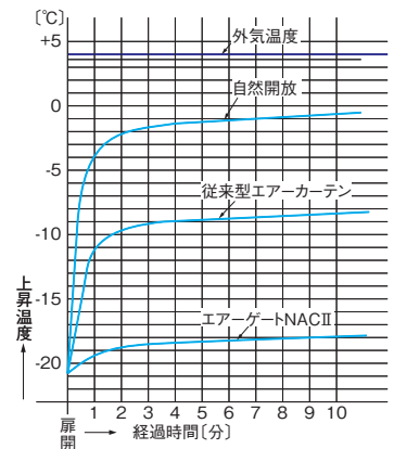
第6図 扉解放時温度上昇グラフ (24ポイント平均)
