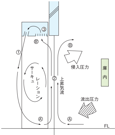
トンネル・サーキュレーション方式
